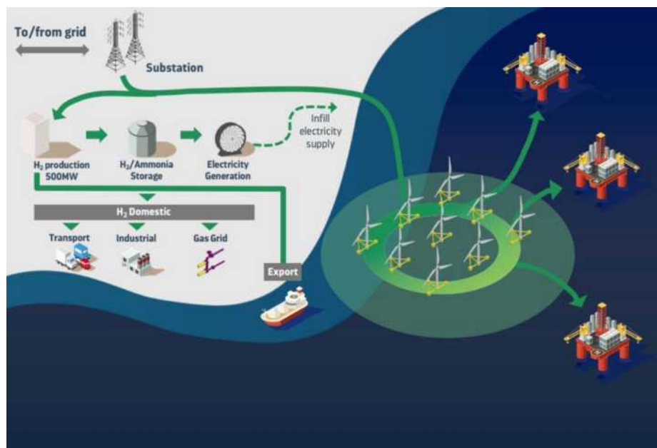
Figura 1. Esquema propuesto en el Reino Unido para reducir la emisión de CO 2 rápidamente, del O&G, con eólico e hidrógeno 2 .
