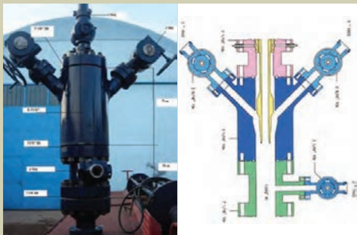
Figure 3. Árbol de Navidad utilizado durante la operación.
