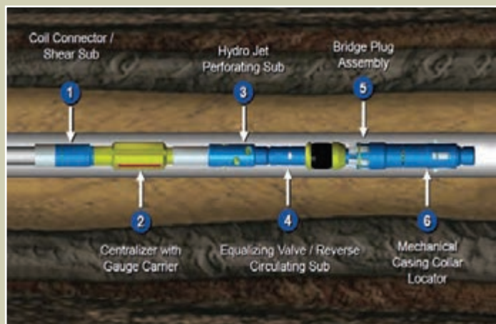
Figure 1. BHA utilizado para realizar las fracturas.
