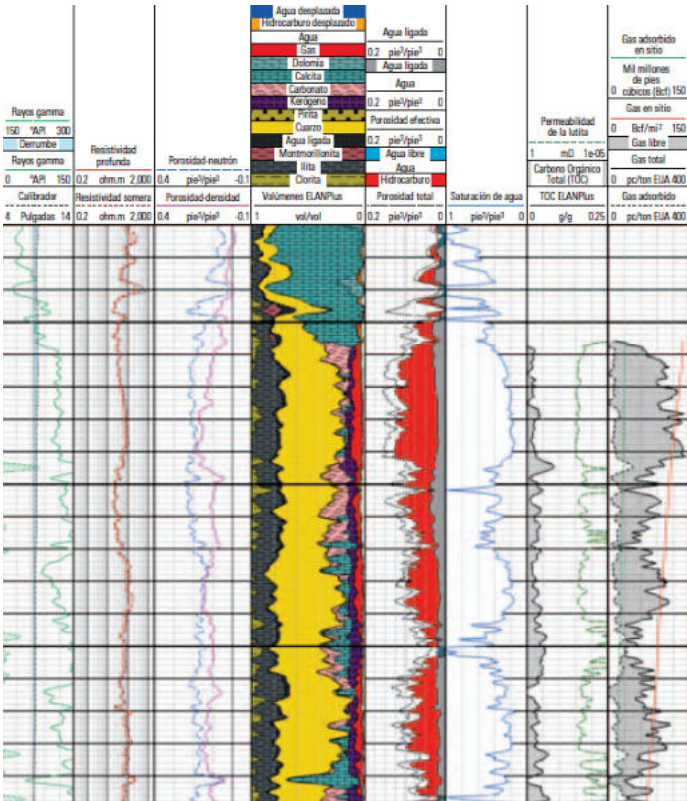
Figura 5: Registros de la Formación Barnett Shale. Los primeros tres carriles presentan las mediciones de la herramienta Platform Express*. El Carril 4 presenta los resultados de un modelo petrofísico generalizado de lutita gasífera, basado en los datos Platform Express* y ECS*, que han sido procesados con el análisis avanzado de registros multiminales ELANPlus. Este programa ayuda a cuantificar la mineralogía, el kerógeno y la porosidad rellena con gas y agua. Los carriles restantes cuantifican la porosidad total y efectiva, la saturación de agua, el contenido TOC, la permeabilidad de la matriz, el gas en sitio y el gas acumulado. Los valores del gas en sitio y el gas acumulado se calculan tanto para el gas libre como para el gas adsorbido.
