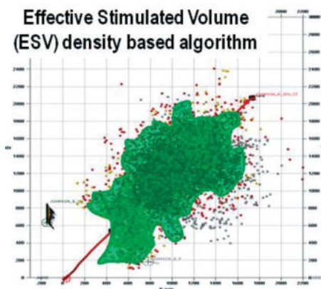
Figura 9: ESV determinado por StimMAP (MAP: Es marca registrada de Schlumberger).
