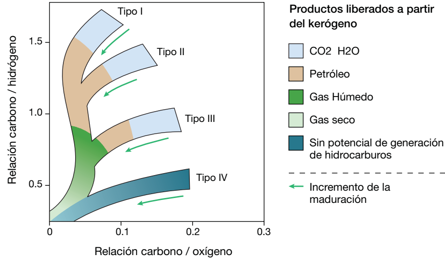
Figura 3: Evolución del kerógeno. (Diagrama de Van Krevelen). Cambios producidos en el kerógeno por el aumento del calor durante el sepultamiento. El kerógeno pierde oxígeno principalmente al emitir CO 2 y H 2 O; luego, comienza a perder más hidrógeno al liberar hidrocarburos.
