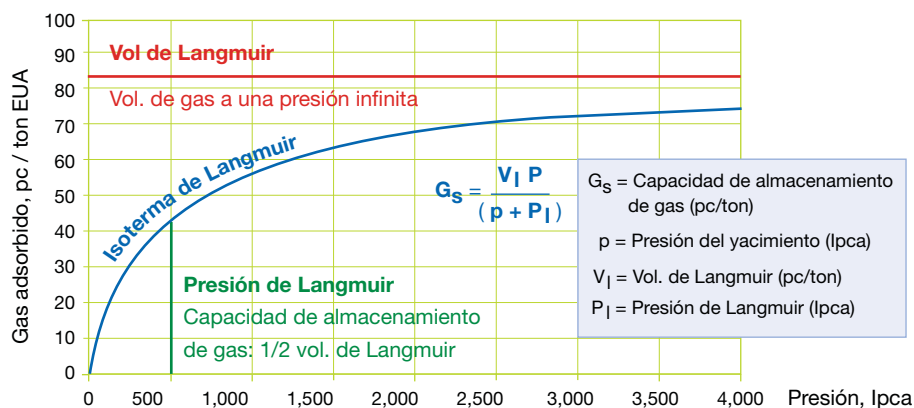
Figura 7: Isoterma de Langmuir.
