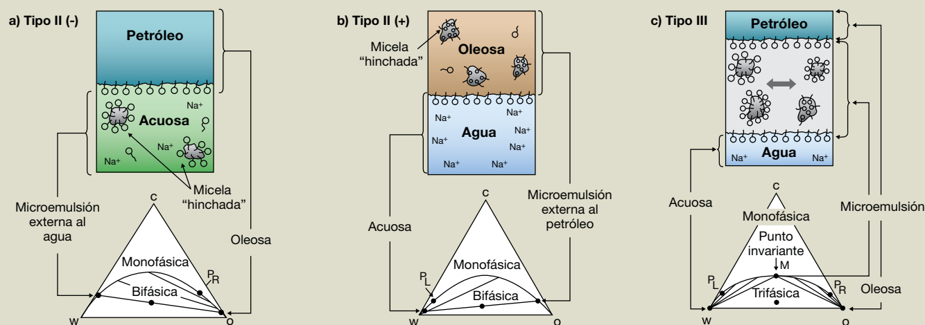
Figura1: Tipos de comportamiento de fase (tomado de Lake, 1989).
