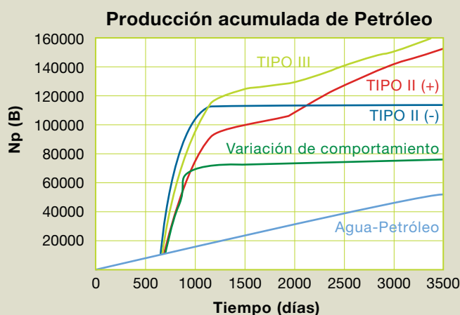
Figura 2: Volumen de petróleo producido acumulado obtenido en los 5 casos testeados.
