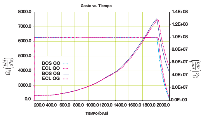
Figura 3 Ritmos de Producción de gas y aceite del pozo productor.
