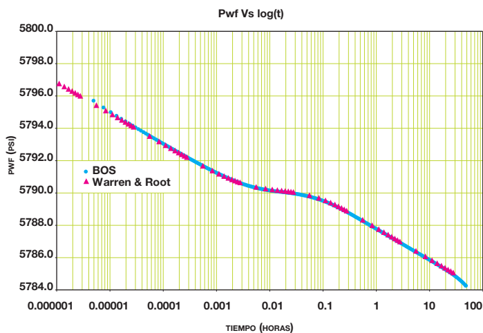
Figura 1: Validación con la solución de Warren&Root
