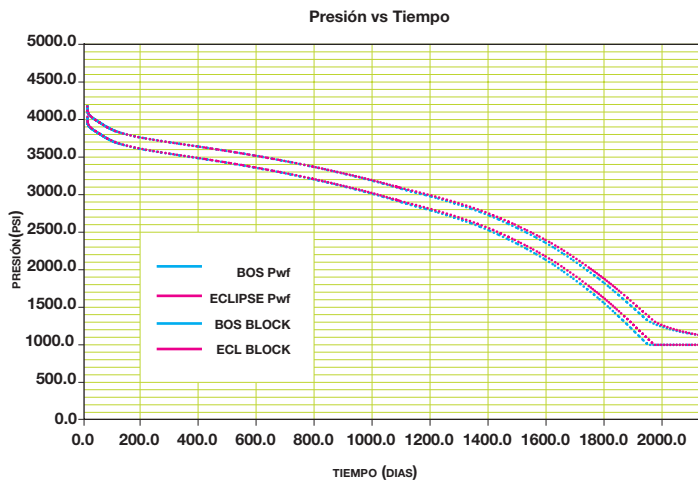
Figura 2: Presión del bloque y de fondo fluendo del pozo productor
