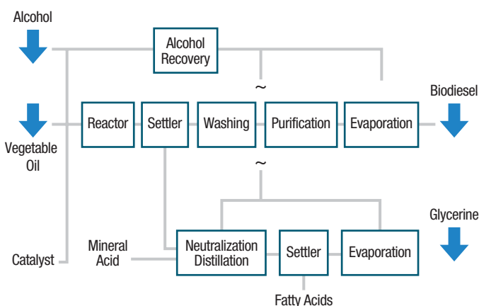
Figura 6: flow sheet de las unidades de producción
