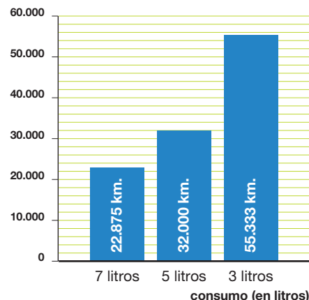
Figura 4: Recorridos con biodiesel, 1.600 litros / ha de cosecha
