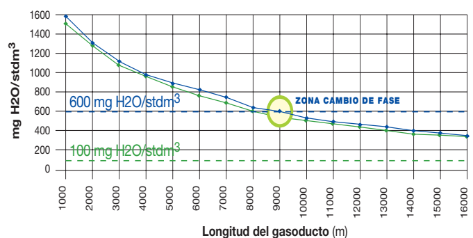
Fig. 2. Concentración de agua en gas
