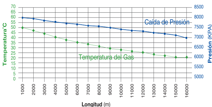
Figura 1. Perfil de temperatura y presión.
