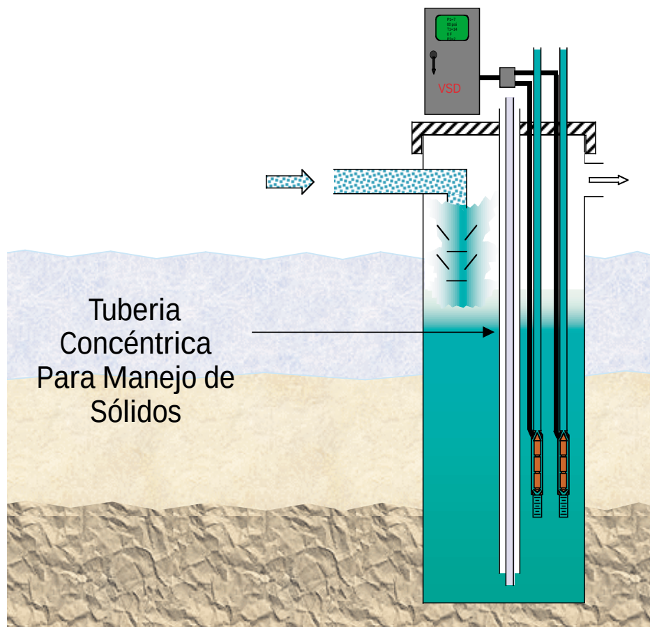
Instalación Sencilla "SIPS-S"
