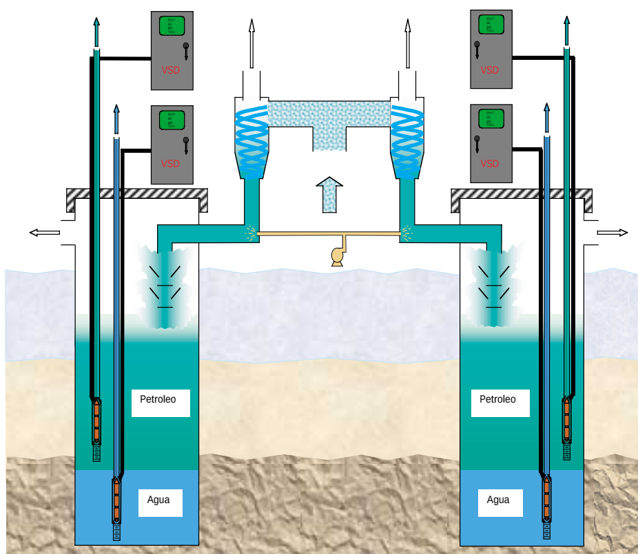
Instalación Múltiple "SIPS-M" - Separación de Agua
